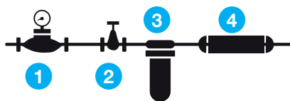
A Standardní zapojení na přívod vody (např. byt)
